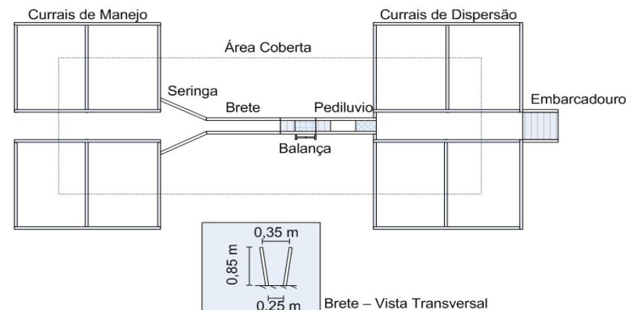
Desenho esquemático - Centro de manejo
